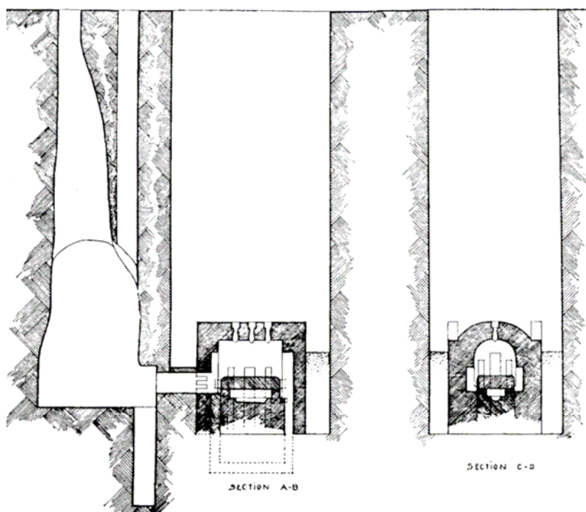
Рис.2 Разрезы гробницы Амена-Тэфнахта
