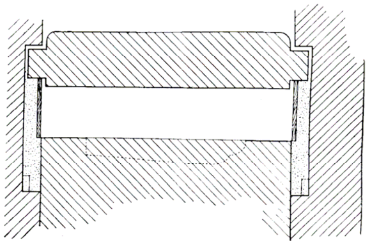
Рис.5 Схема работы «опускного механизма» крышки известнякового саркофага.
